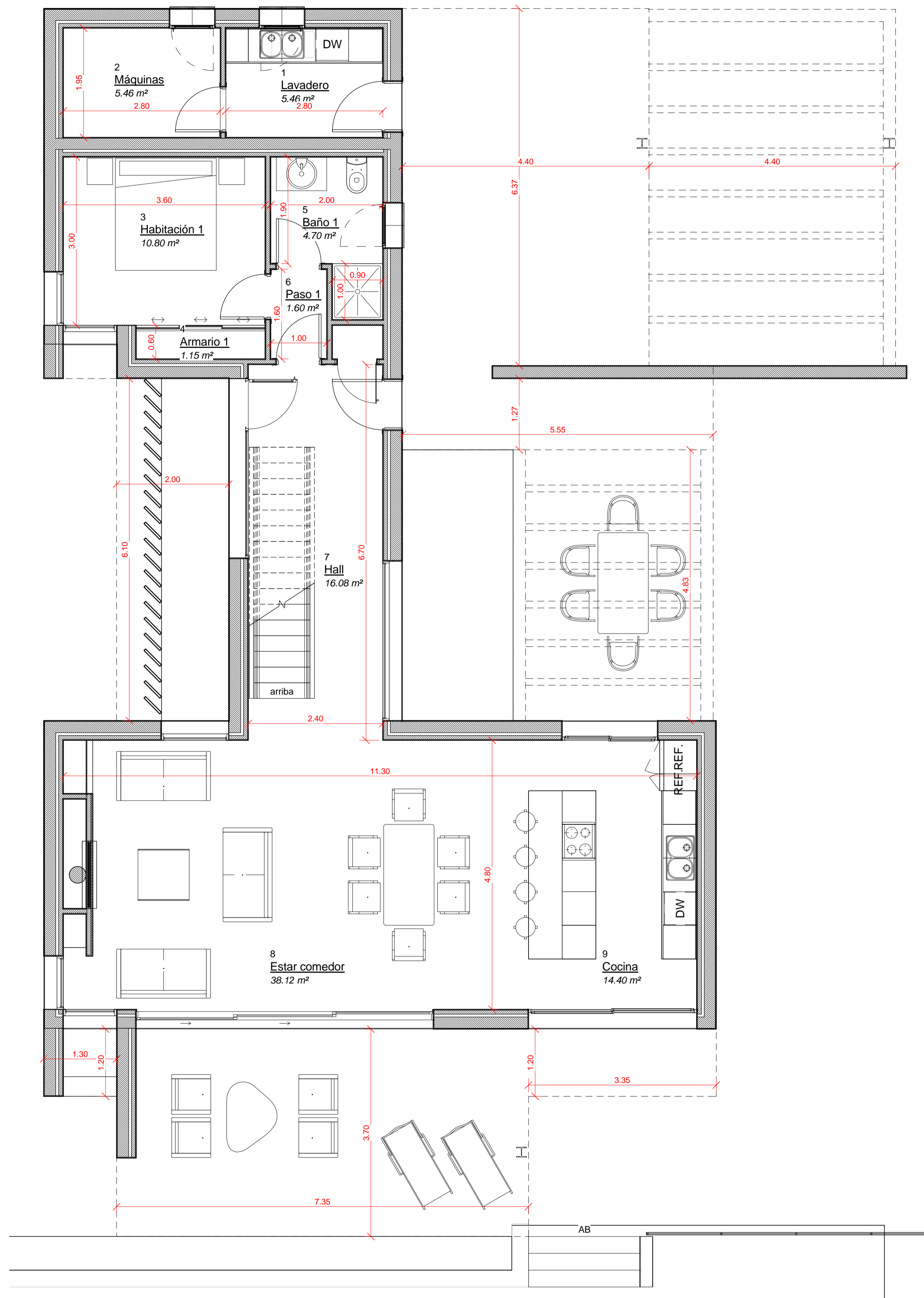
1 Nivel 1 cotas A103 1:50
